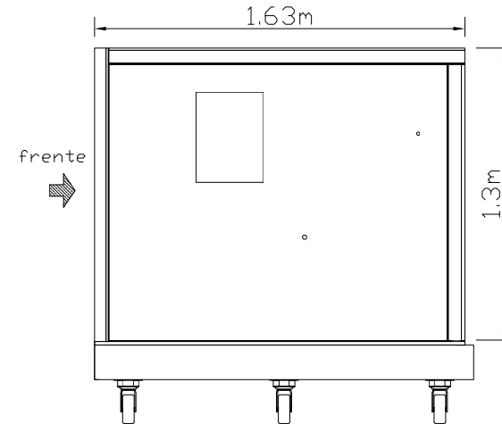
VISTA LATERAL DERECHO MF 500-6S
